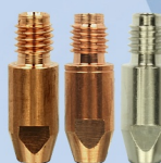
Stromdüse M8 x 30 Art.-Nr. 830□001 Art.-Nr. 830□401 (CuCrZr) Art.-Nr. 830□301 (vernickelt) □ Bitte Drahtstärke eintragen
